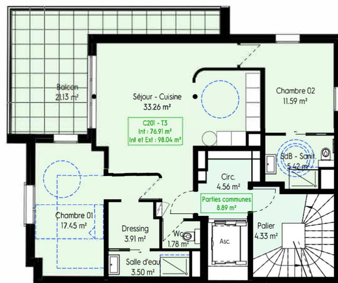
BATIMENT C - 2EME ETAGE
