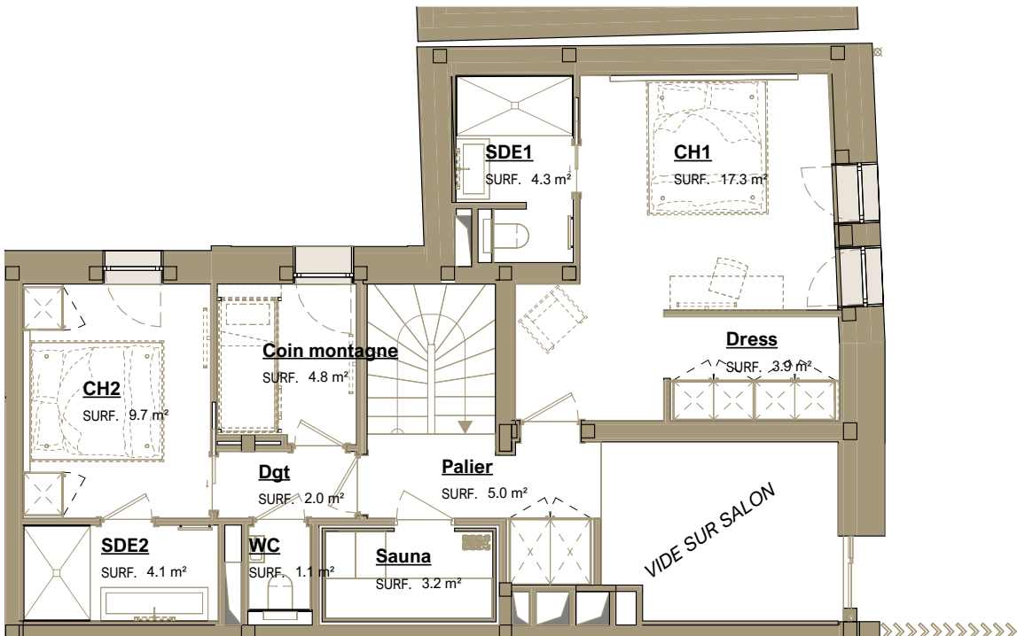
02_R+1 1 : 100
