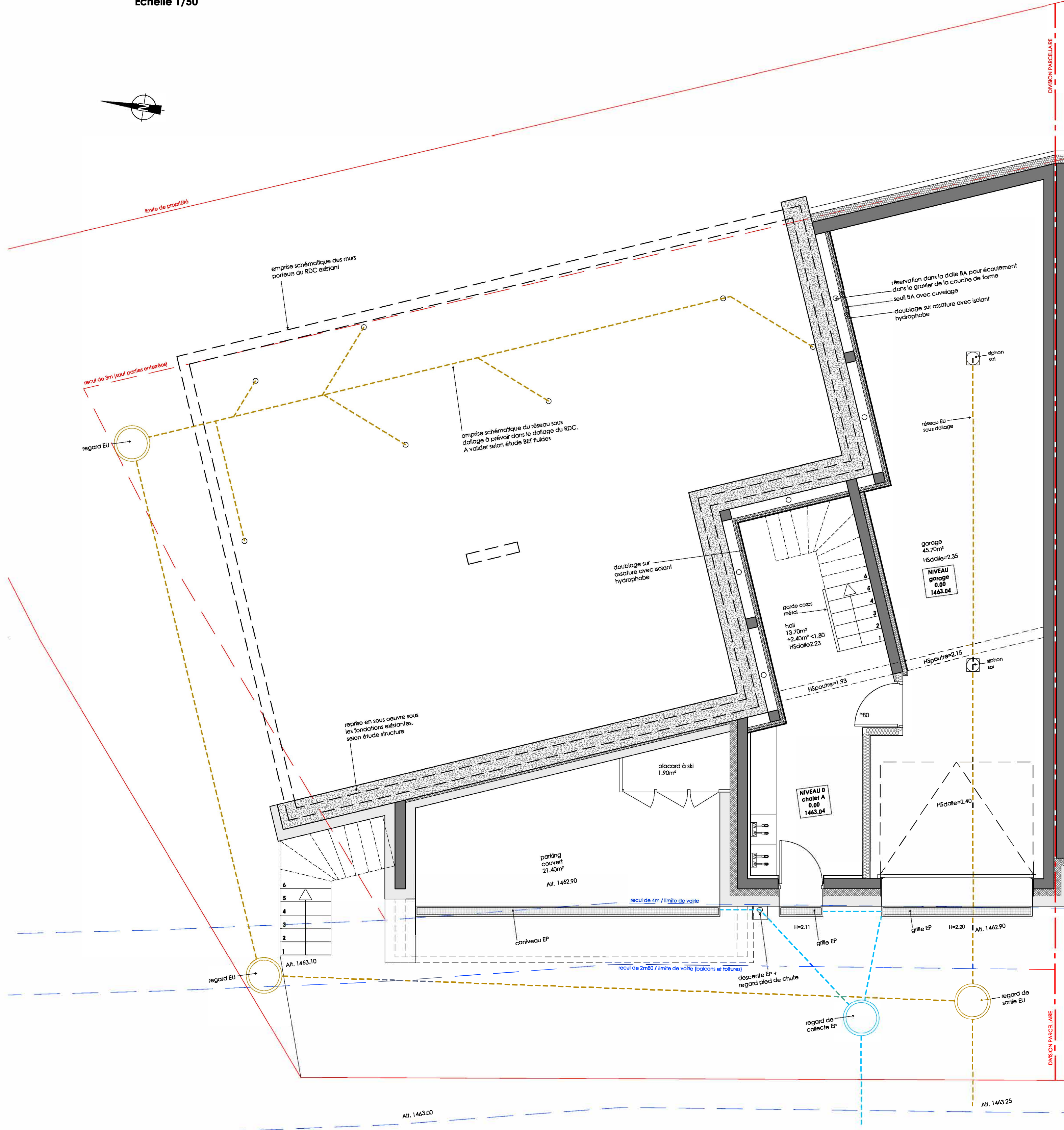
Plan Niveau 0 / chalet A Echelle 1/50
